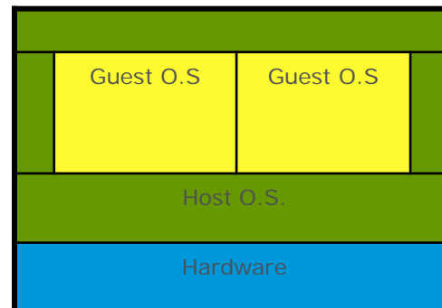
OS-Level Virtualisation
